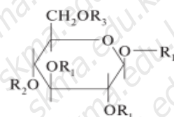
Китайский танин
