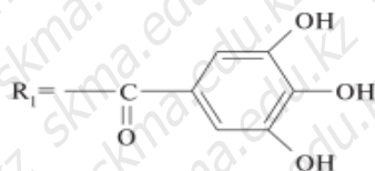
Галловая кислота
