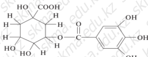
Теогаллин (депсид)
